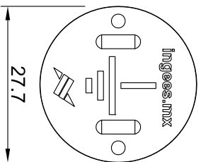
VISTA SUPERIOR DE TAPA
