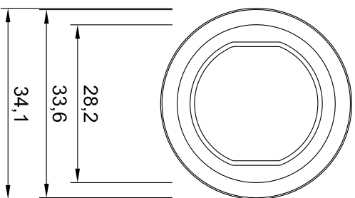
VISTA SUPERIOR DE ARO
