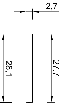
VISTA FRONTAL DE TAPA
