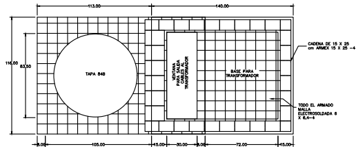
PLANTA BASE PARA TRANSFORMADOR Y REGISTRO TIPO 3 EN BANQUETA
