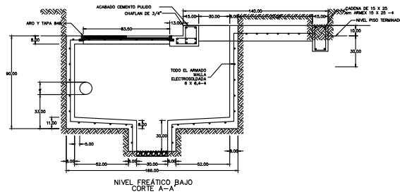
NIVEL FREÁTICO BAJO CORTE A-A'
