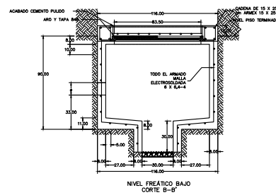
NIVEL FREÁTICO BAJO CORTE B-B'
