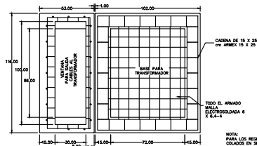
PLANTA BASE PARA TRANSFORMADOR CUANDO SE FABRICA INDEPENDIENTE DEL REGISTRO
