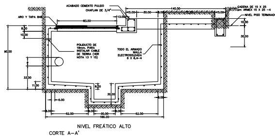
NIVEL FREÁTICO ALTO CORTE A-A'
